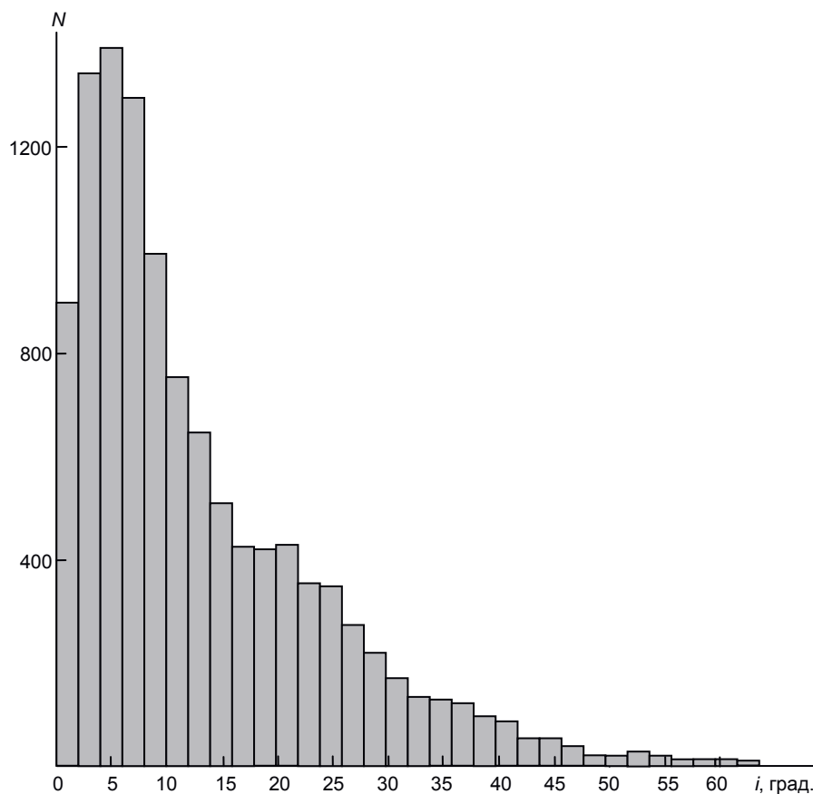
Рисунок 3. Распределение астероидов по наклону к плоскости эклиптики. Figure 3. The distribution of asteroids in inclination to the ecliptic plane.
