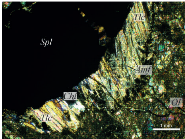
Figure 2. The development of talc Tlc , chromic clinocllore Chl , serpentine Srp and tremolite Amf in pressure shadows at the nodule border of chrome-spinel Spl with serpentinized olivine Ol . Thin section photo in cross-polarized light. Рисунок 2. Развитие талька Tlc , хромового клинохлора Chl , серпентина Srp и тремолита Amf в тенях давления на границе нодуля хромовой шпинели Spl с серпентинизированным оливином Ol . Фото шлифа с анализатором.
