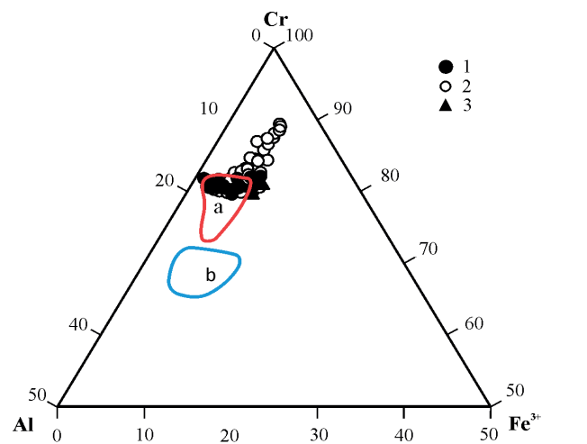
Figure 4. The compositions of ore-forming chrome-spinels from nodular chromite ores of the Engayskoe-3 occurrence. 1 – nodule rim; 2 – nodule core; 3 – chrome-spinel impregnation in the space between the nodules; a, b – fields of ore-forming chrome-spinel compositions according to [10]: a – Tsentralnoye deposit, b – Engayskoe-1 occurrence. Рисунок 4. Составы рудообразующих хромовых шпинелей из нодулярных хромититов рудопоявления Енгайское-3. 1 – кайма нодуля; 2 – ядро нодуля; 3 – вкрапленность хромовой шпинели в пространстве между нодулями; а, б – поля составов рудообразующих хромовых шпинелей по [10]: а – месторождение Центральное, б – рудопоявление Енгайское-1.
